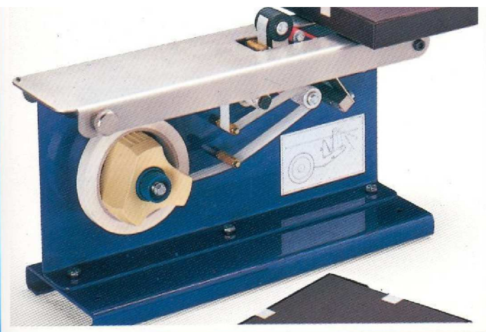
C19 ANGOLATORE ● L-CLIP SEALER ● DEVIDOIR MANUELL POUR POSE ONGLETS ● KANTENSCHLISSER ● ANGULADOR
